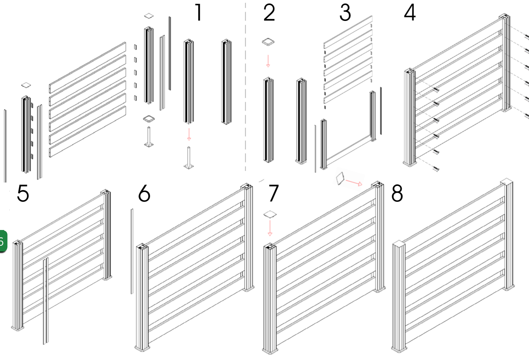
Dikey GoldFence Montajı
